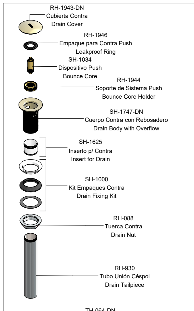
Contra de Push para Lavabo con Rebosadero Lavatory Sink Pop-up Drain with Overflow
